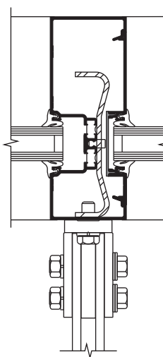
MONTANT DU 601UT
