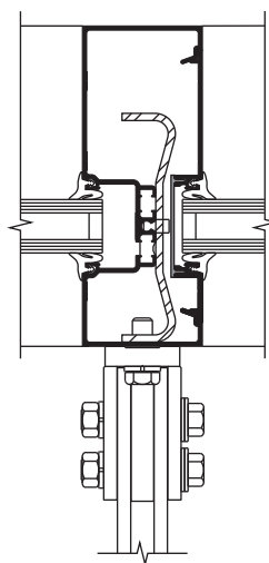
MONTANT DU 601T
