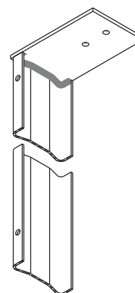
ANCRAGE DE TÊTE POUR CADRES À ASSEMBLAGE À VIS ET CANNELURES
