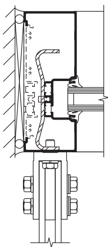
JAMBAGE TRIFAB® 601T (TF 601 ET 601UT SIMILAIRE)
