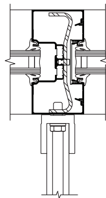
MONTANT DU 451UT
