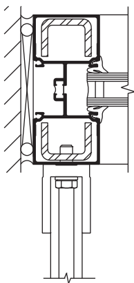
JAMBAGE TRIFAB® VG 451T (TF VG 451 SIMILAIRE)
