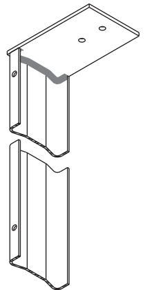
ANCRAGE DE TÊTE POUR CADRES À ASSEMBLAGE À VIS ET CANNELURES
