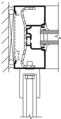
JAMBAGE TRIFAB® VG 451T (TF VG 451 ET 451UT SIMILAIRE)
