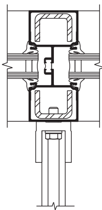
MONTANT DU 451T
