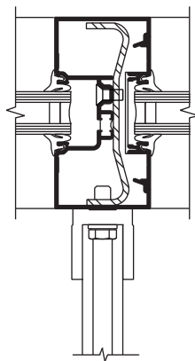
MONTANT DU 451T
