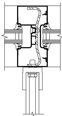
MONTANT DU 451
